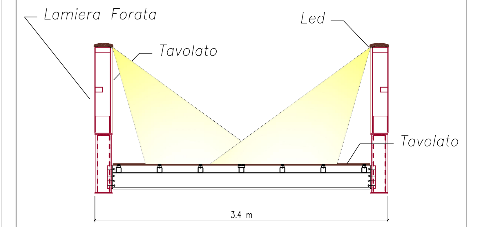
SEZIONE IN MEZZERIA Scala 1:25
