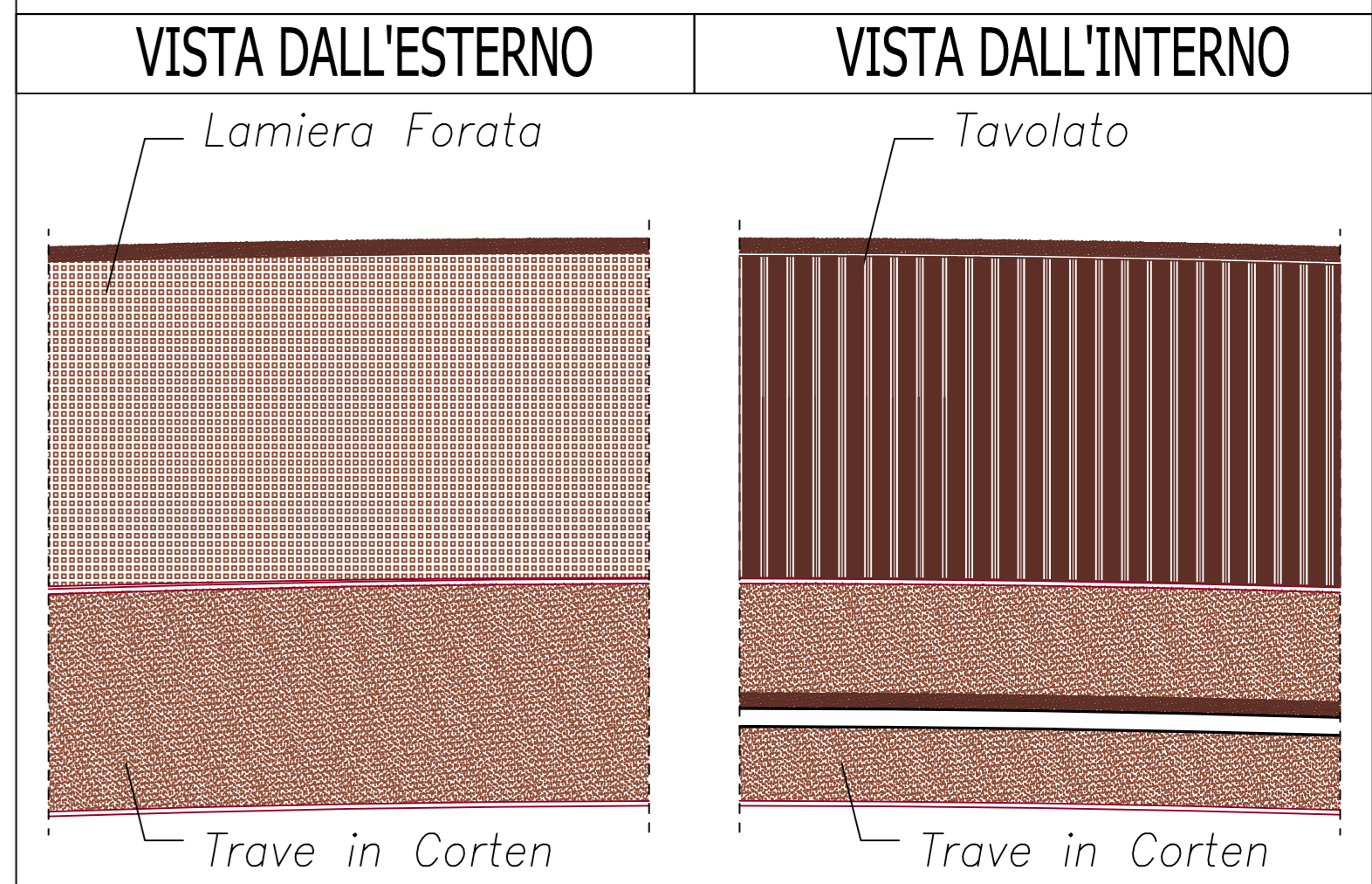
DETTAGLIO DEL PARAPETTO Scala 1:20
