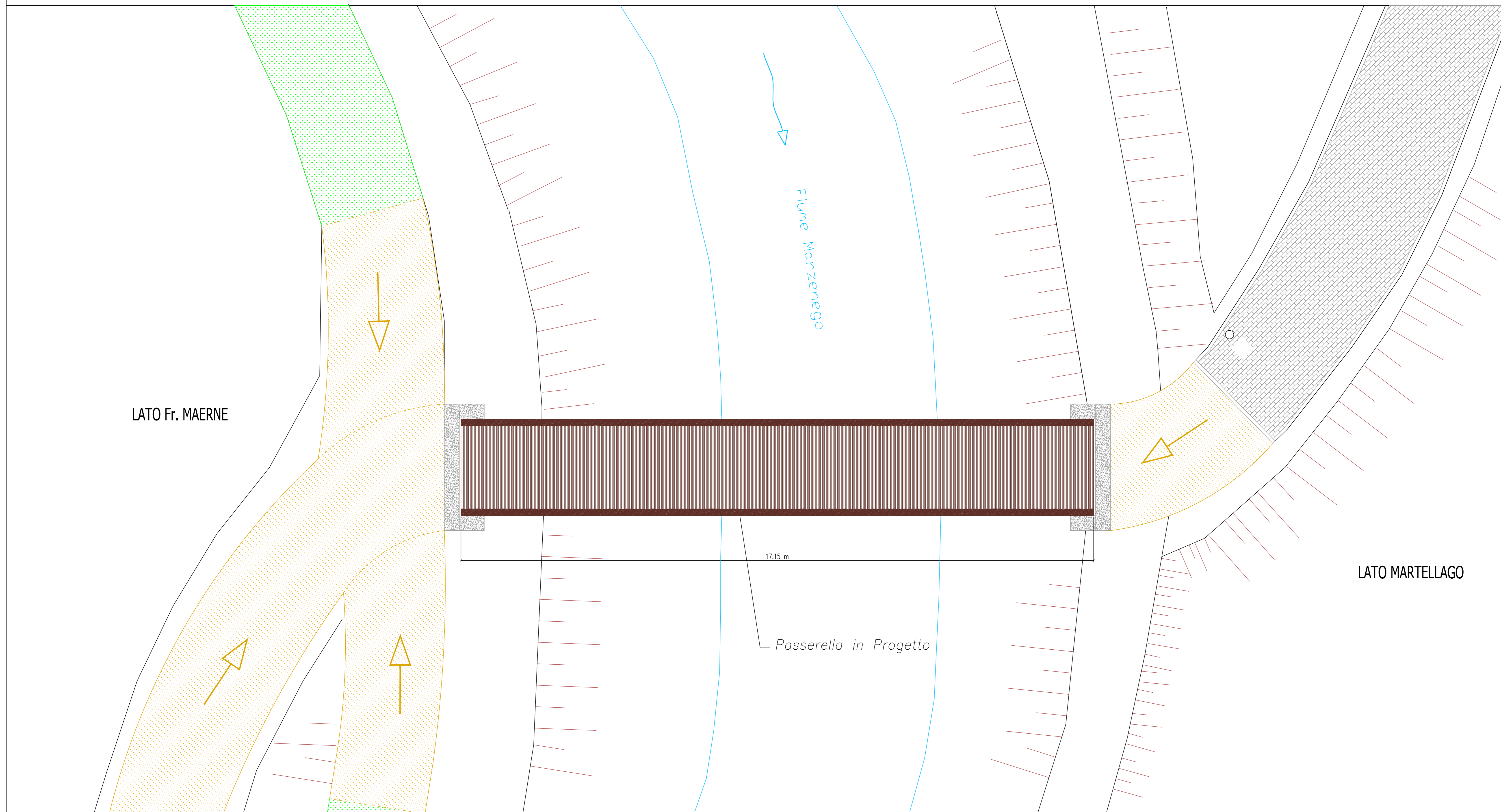
PIANTA DELLA PASSERELLA Scala 1:50
