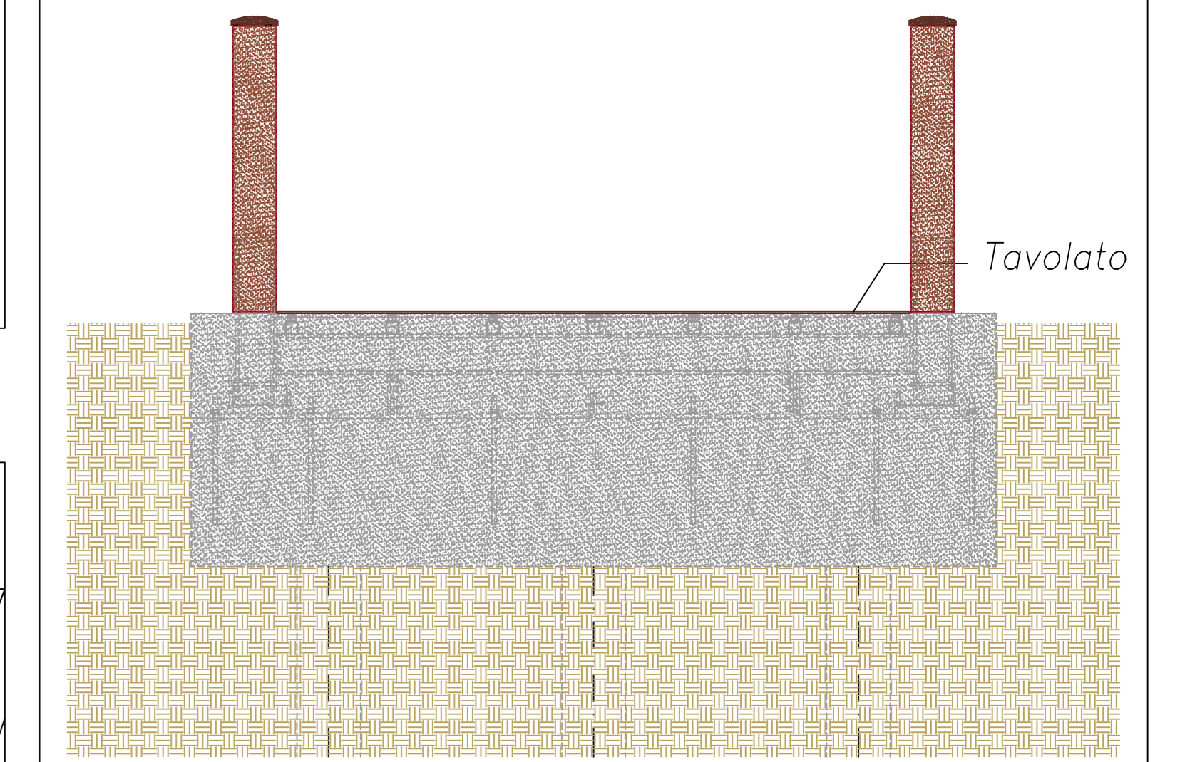
SEZIONE IN APPOGGIO Scala 1:25
