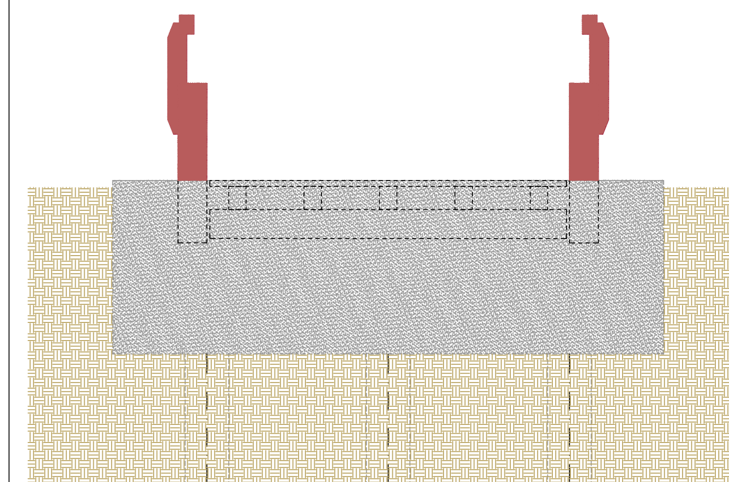
SEZIONE IN APPOGGIO Scala 1:25
